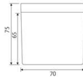
スライドポケット正面図
