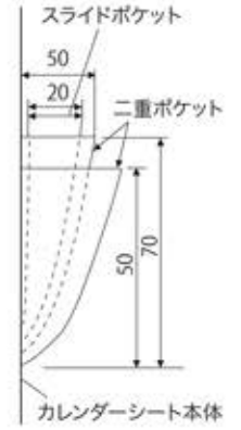
ポケット収まり図(側面)
